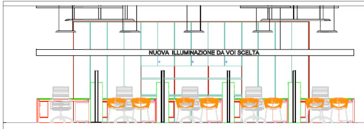
PROSPETTO UFFICIO ANAGRAFE - URP
