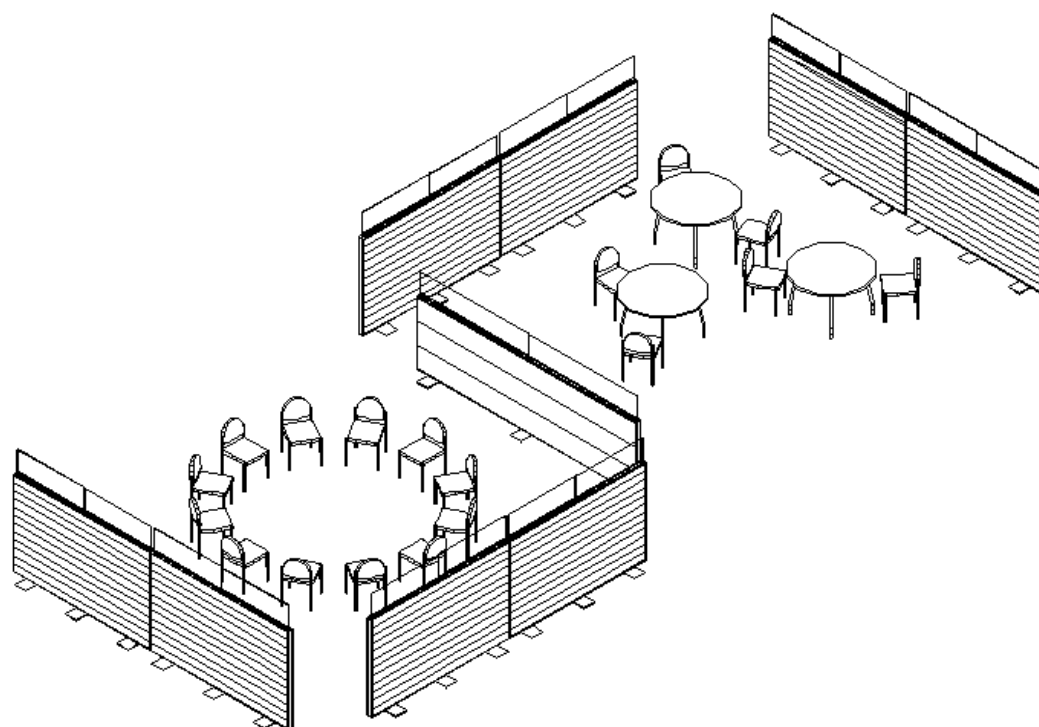
Ipotesi con Acoustic Open Space \alpha -Floor \alpha -Desk in un asilo
