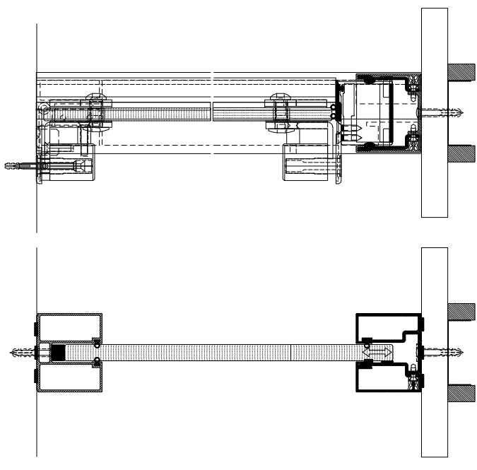
SEZIONE PARETI SCALA 1:2
