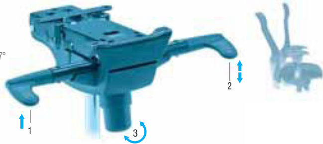
Synchron + Traslatore + Varia (Variatore angolo sedile-schienale) (mod. Kubika + Kamelia) Synchron + Slide System + Varia (Seat-back angle adjustment) (mod. Kubika + Kamelia) (inclinazione negativa/Negative inclination -3°)
