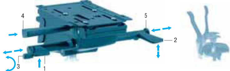
Synchron + Traslatore + Varia (Variatore angolo sedile-schienale) (mod. Kubika + Kamelia) Synchron + Slide System + Varia (Seat-back angle adjustment) (mod. Kubika + Kamelia) (inclinazione negativa/Negative inclination -3°)
